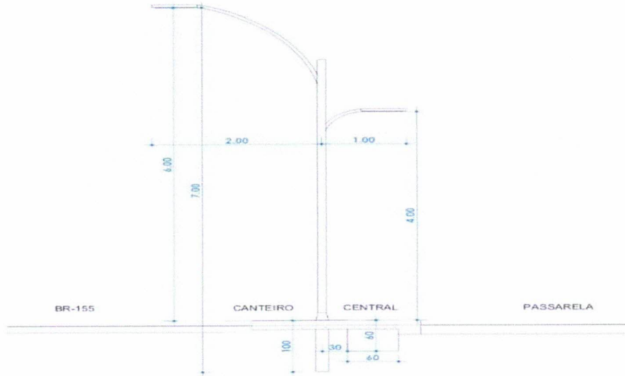
DETALHES DO POSTE SEM ESCALA
