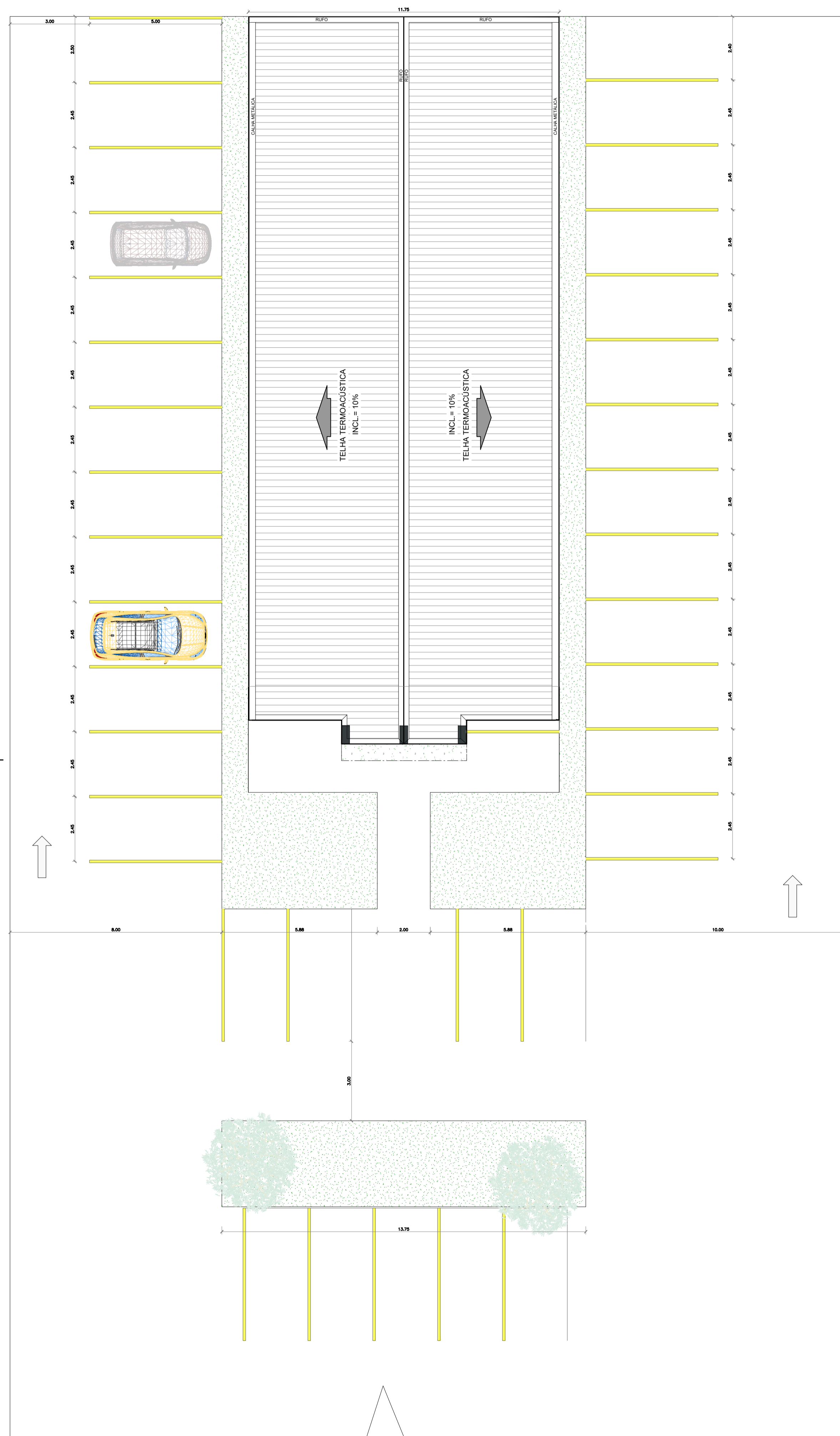
1 PLANTA DE COBERTURA E LOCAÇÃO ESCALA 1:100
