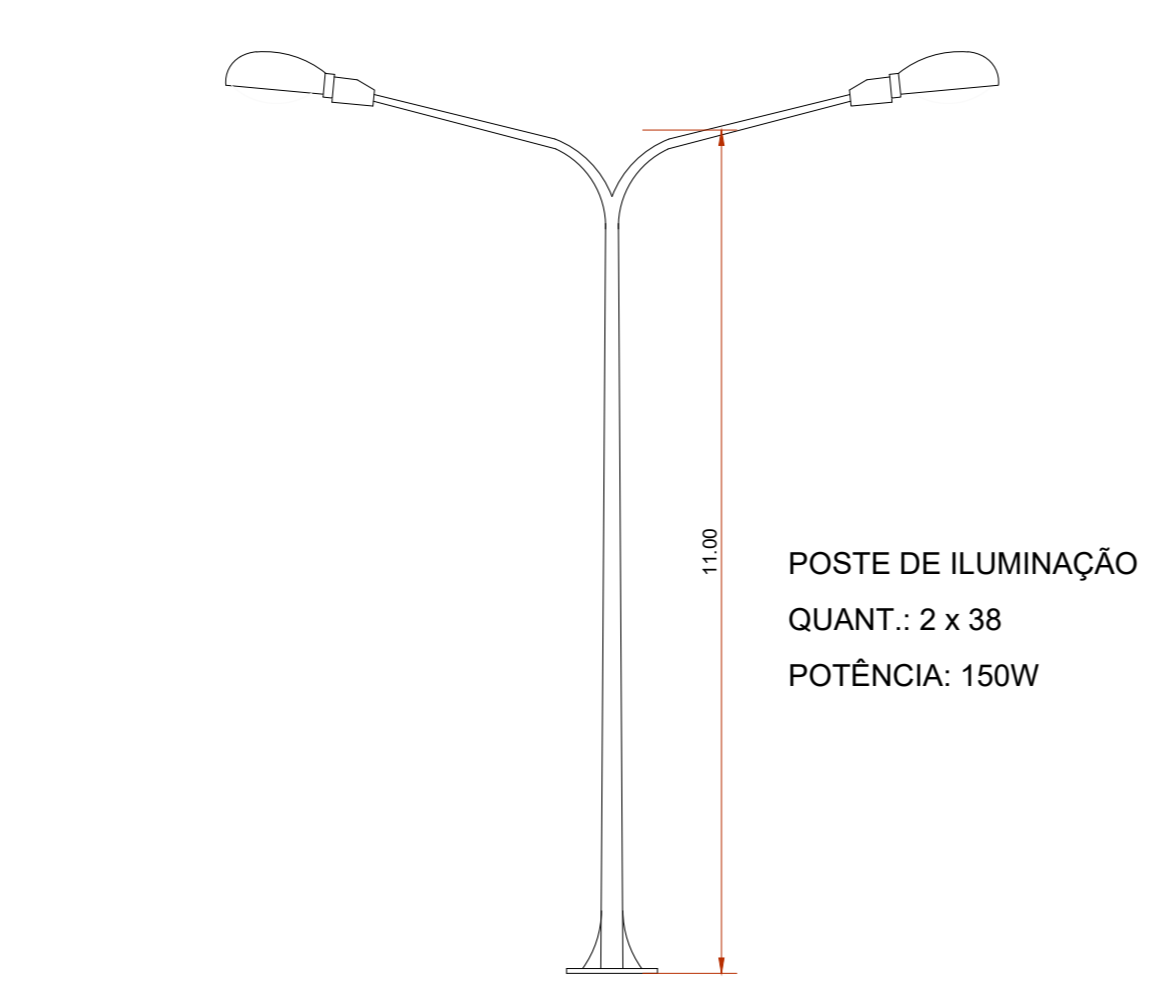
5 DETALHAMENTO DE POSTE DE ILUMINAÇÃO SEM ESCALA
